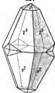
Calcite.
